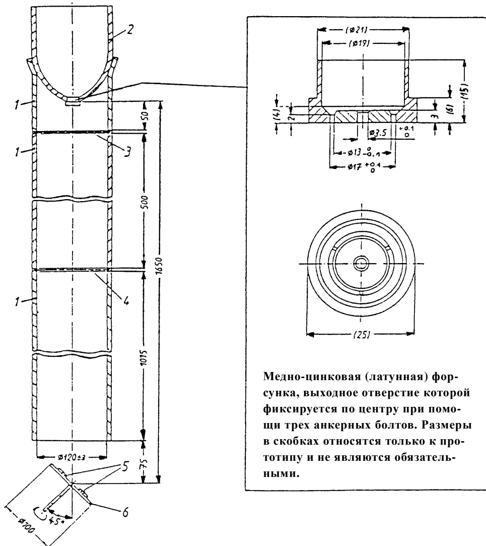
Рис. 6 Устройство для испытания под струей песка
