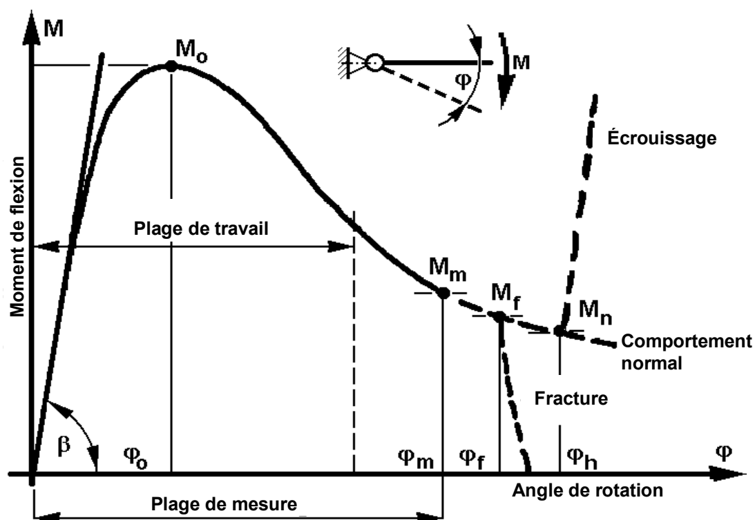
Figure A8.A1.1 – Courbe caractéristique d'une articulation plastique
