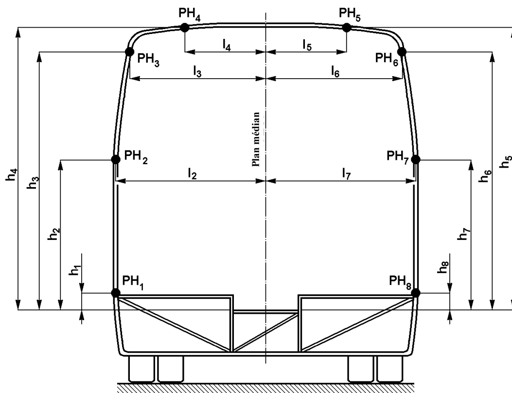
Figure A8.1 – Paramètres géométriques des articulations plastiques d'un segment
