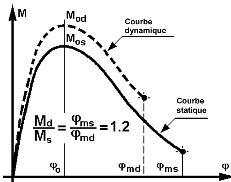
Figure A8.A1.2 – Courbe dynamique déduite de la courbe statique pour une articulation plastique
