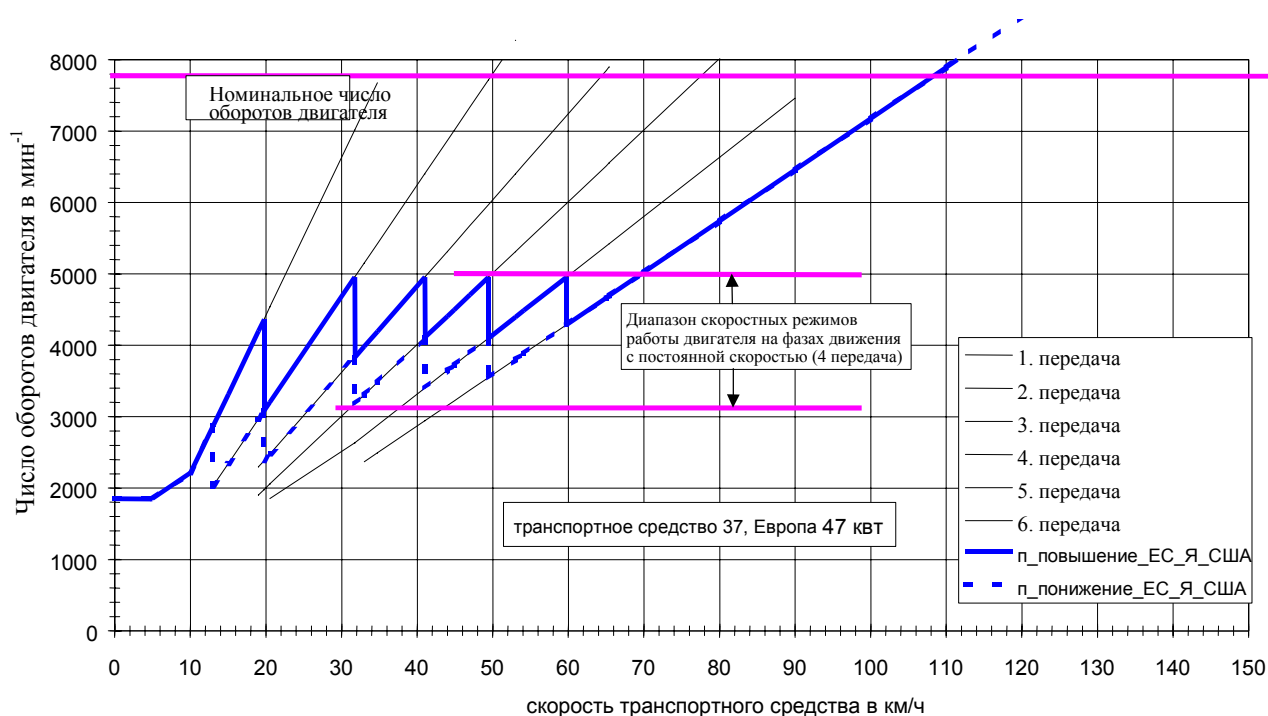
Рис. А13-1: Пример схемы переключения передач легкого транспортного средства
