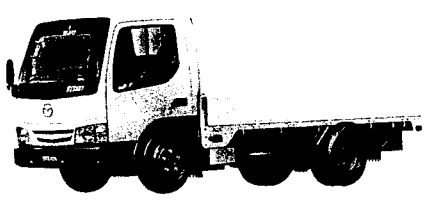
7 タイタン1.5t 3.0ℓ ワイドロー 標準キャビンハイルーフ 標準ボディ デラックス TITAN 1.5 ton 3.0 liter Wide & Low, Narrow Cabin
