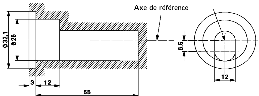
Figure 6 – Dimensions maximales de la lampe 2/
