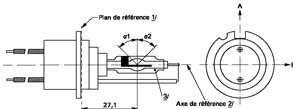
Figure 1 – Catégorie D1R – Type à fils – Culot PK32d-3
