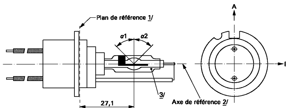
Figure 1 – Catégorie D1S – Type à fils – Culot PK32d-2
