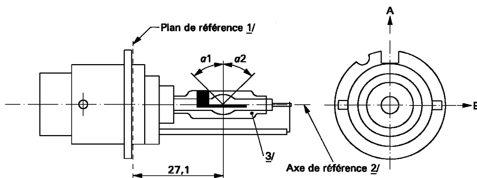
Figure 4 – Catégorie D4S – Type à broche – Culot P32d-5
