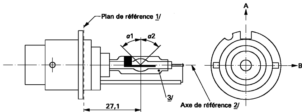
Figure 4 – Catégorie D4R – Type à broche – Culot P32d-6
