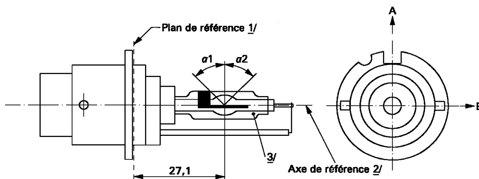
Figure 2 – Catégorie D2R – Type à broche – Culot P32d-3
