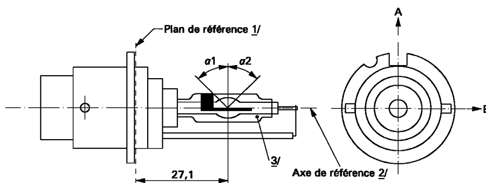
Figure 2 – Catégorie D2S – Type à broche – Culot P32d-2
