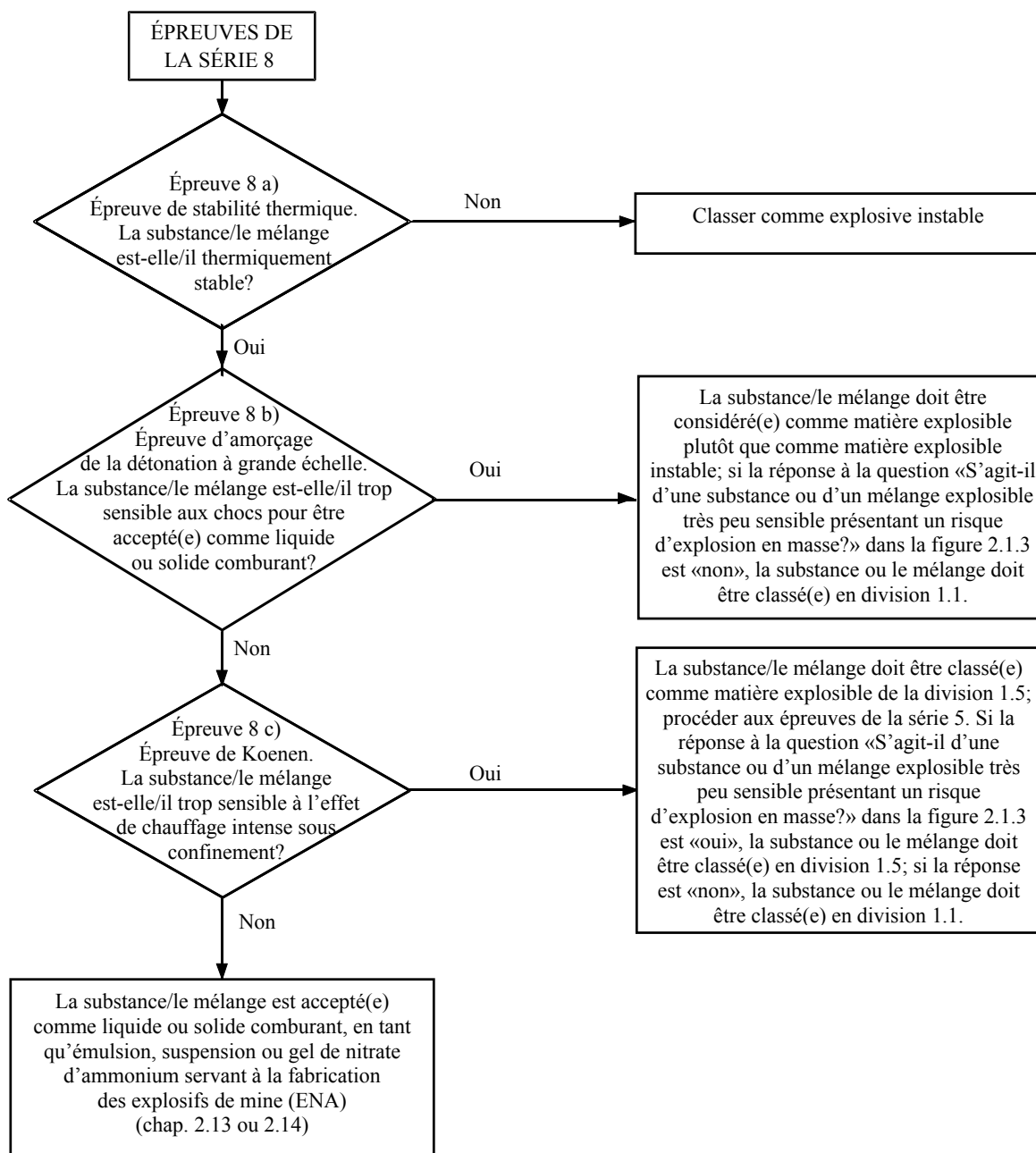
Figure 2.1.4: Procédure pour la classification des émulsions, suspensions ou gels de nitrate d'ammonium
