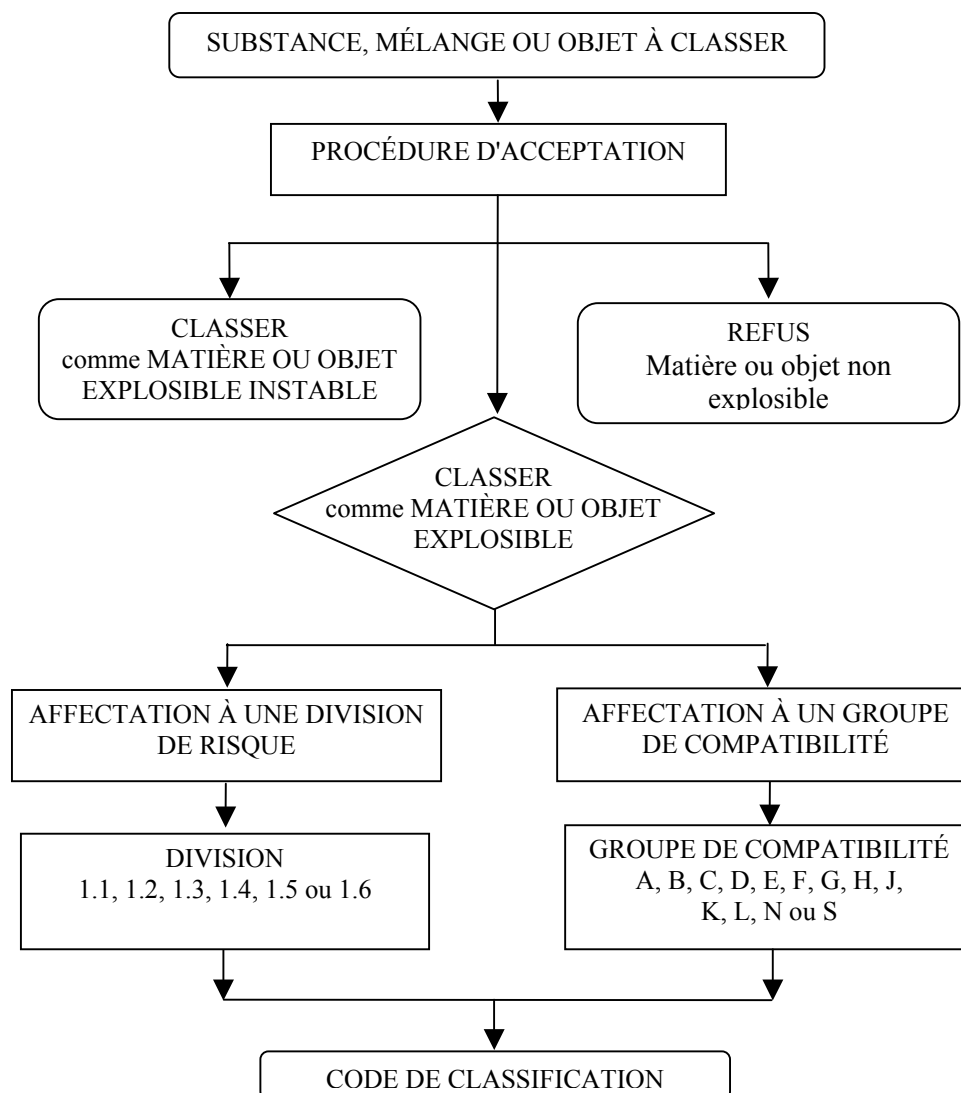
Figure 2.1.1: Diagramme d'ensemble de la procédure de classification d'une substance, d'un mélange ou d'un objet dans la classe des matières et objets explosibles (Classe 1 pour le transport)
