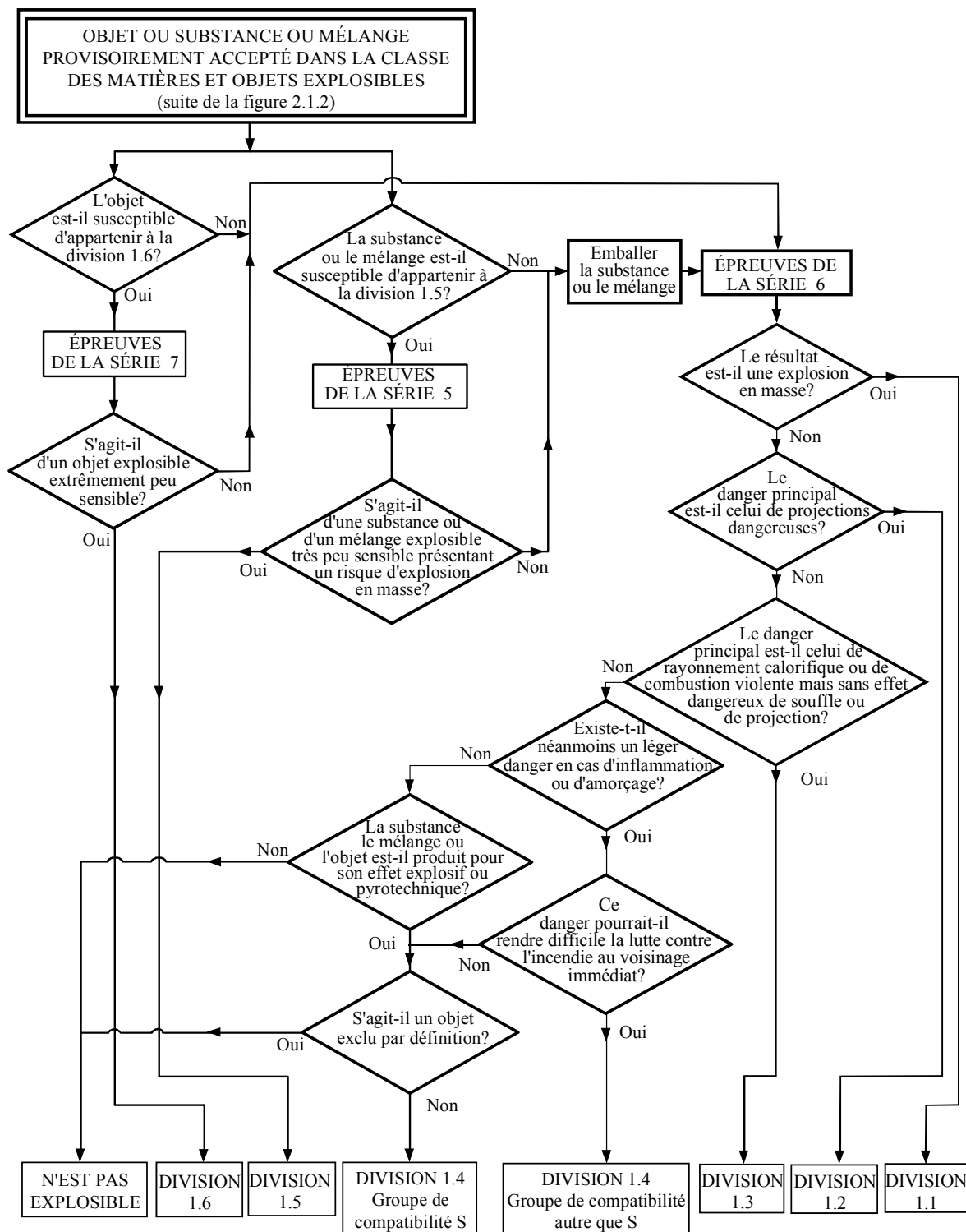
Figure 2.1.3: Procédure d'affectation à une division de la classe des matières et objets explosibles (Classe 1 pour le transport)
