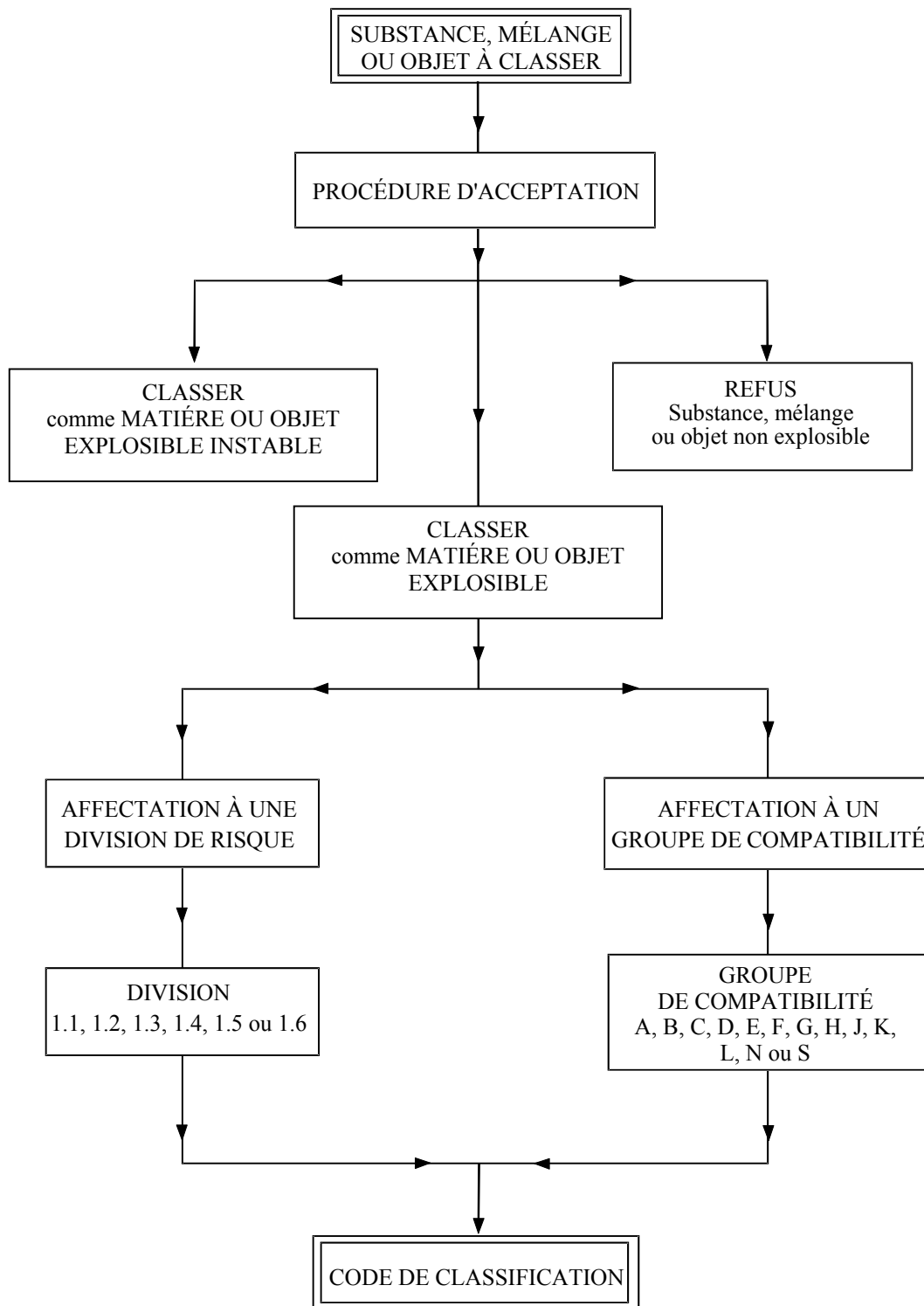
Figure 2.1.1: Diagramme d'ensemble de la procédure de classification d'une substance, d'un mélange ou d'un objet dans la classe des matières et objets explosibles (Classe 1 pour le transport)
