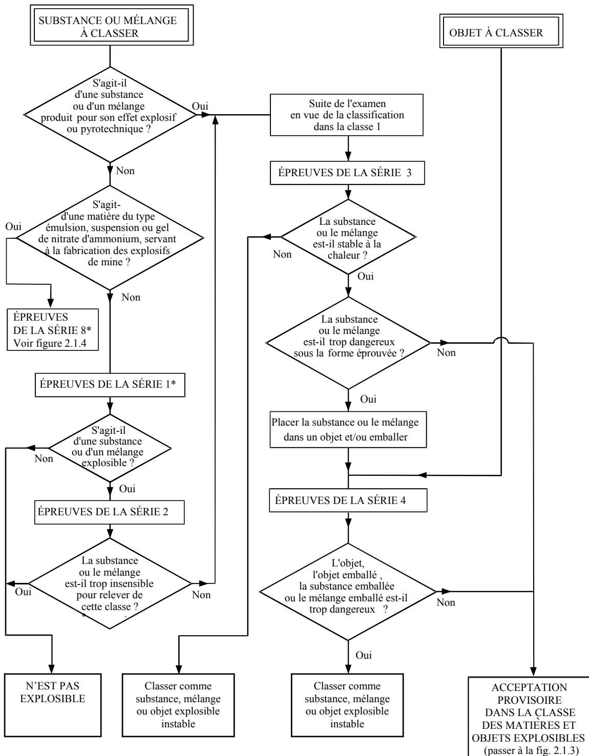
Figure 2.1.2: Procédure d'acceptation temporaire d'une substance, d'un mélange ou d'un objet dans la classe des matières et objets explosibles (Classe 1 pour le transport)
