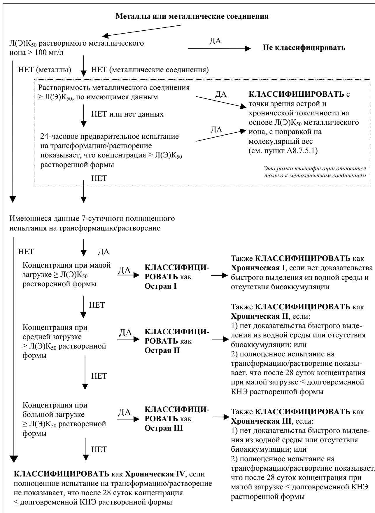
Рисунок А8.7.1: Стратегия классификации металлов и металлических соединений
