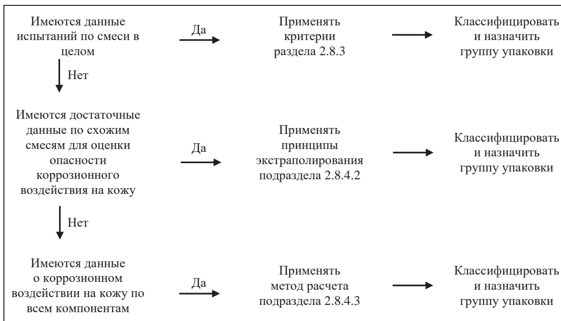
Рис. 2.8.4.1: Поэтапный подход к классификации коррозионных смесей и назначению им групп упаковки
